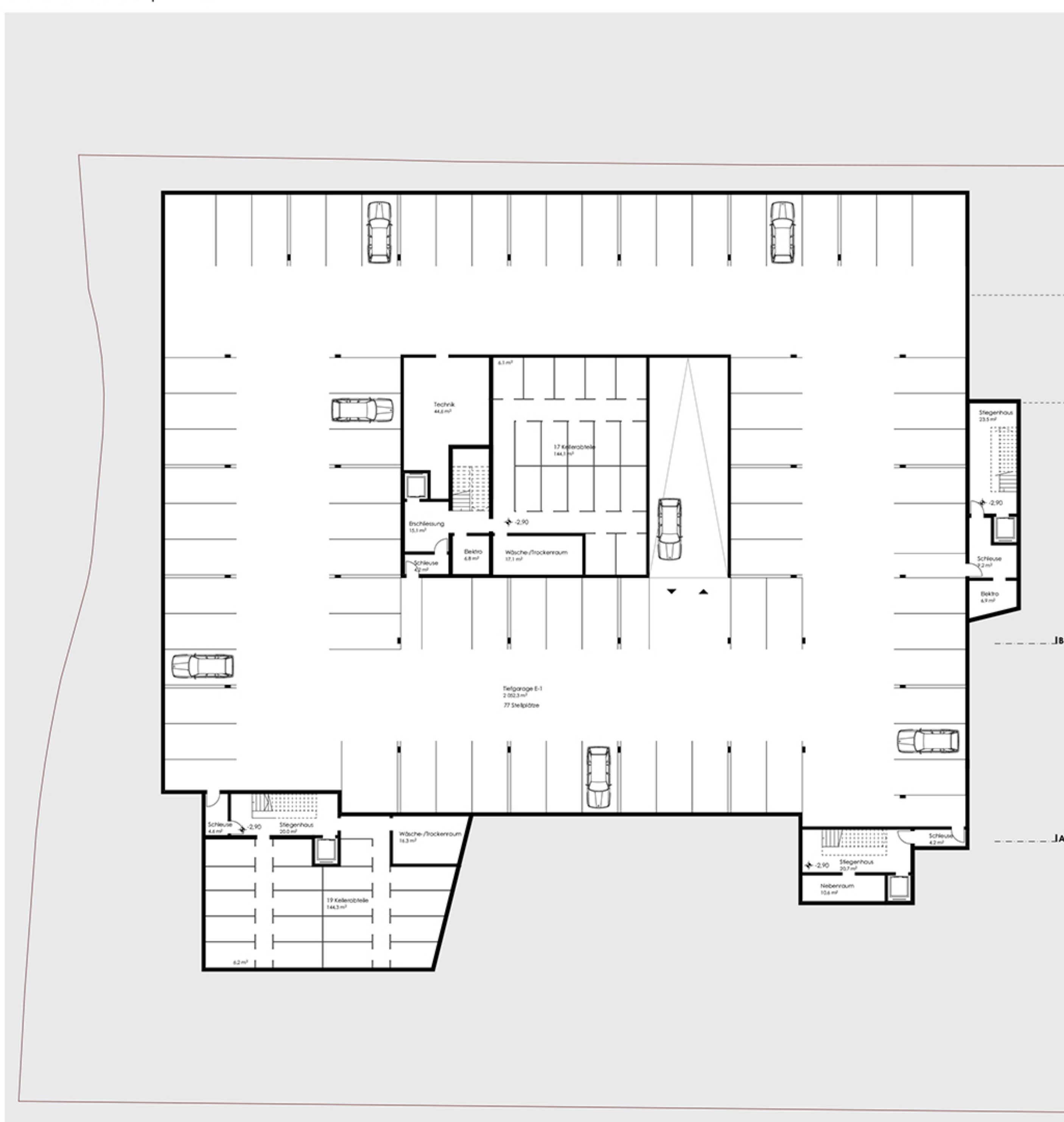
Grundriss Ebene -1 | 1 : 200
