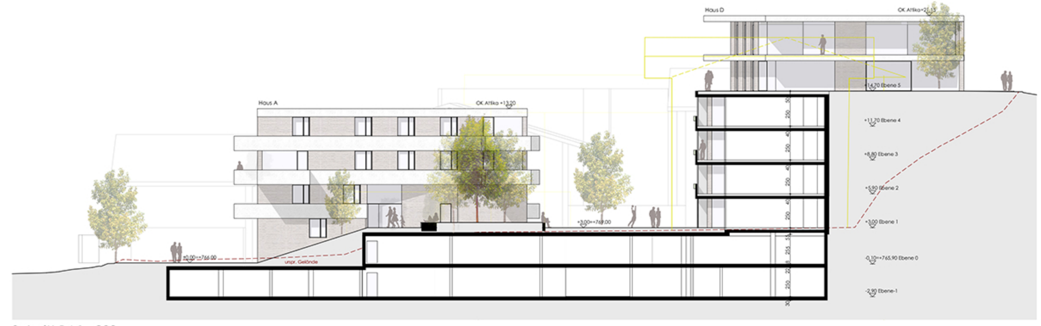
Schnitt B I | 200
